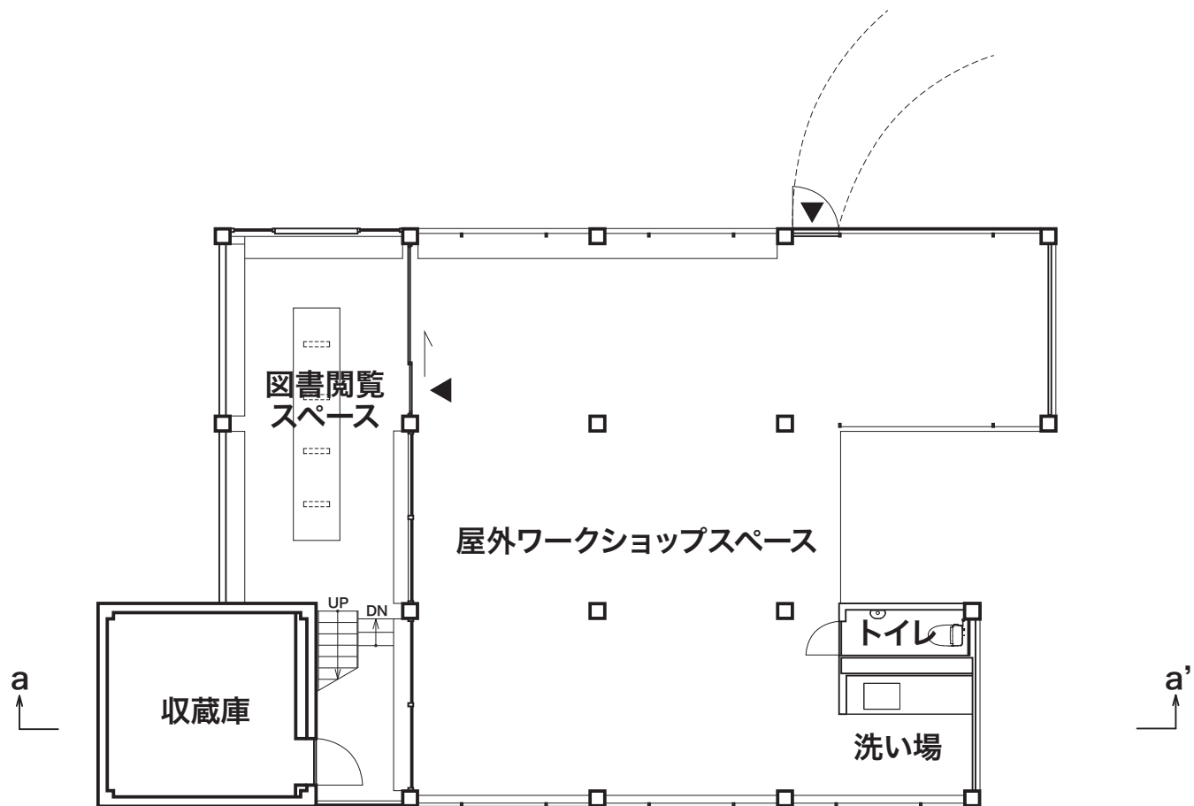
1階平面図
