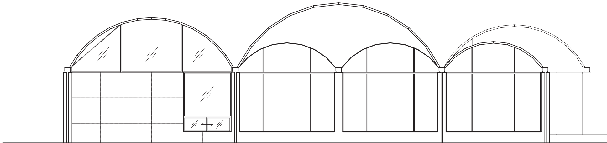
西側立面図
